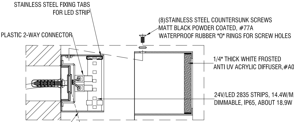
A - A
